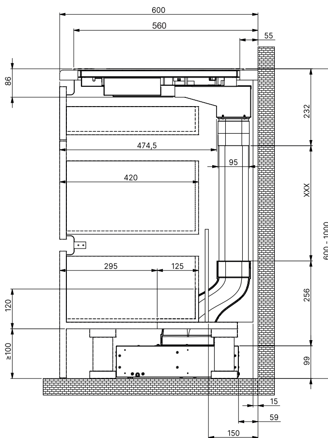
Installatie van zijdelings luchtafvoersysteem
