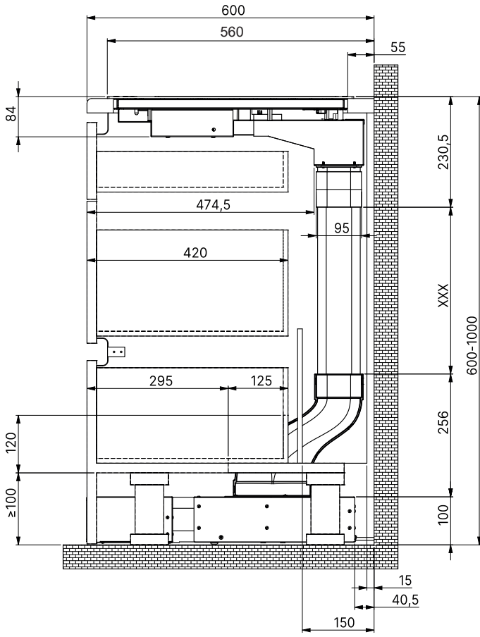
Einbau Umluft mit Gitterblende für Sockelleiste
