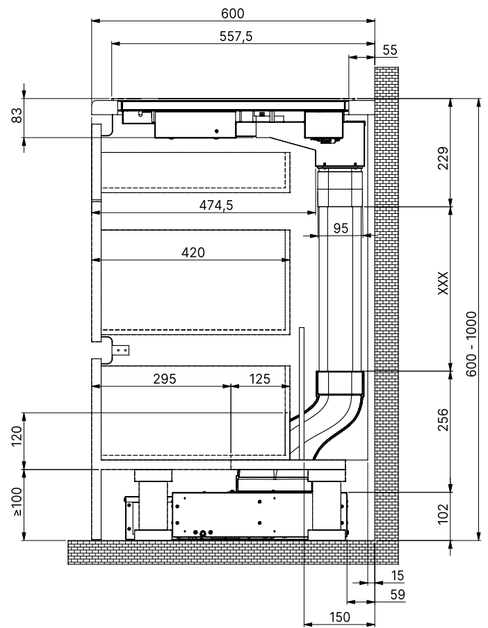
Einbau Umluft mit Kohlefilter im Sockel
