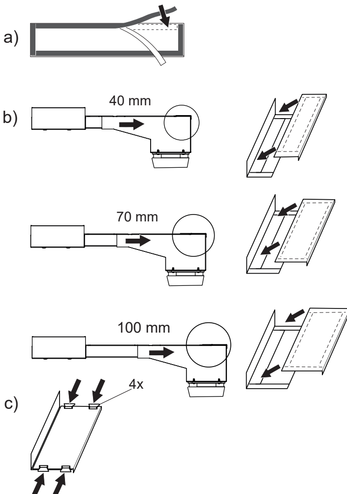
Einbau Umluft mit Gitterblende für Sockelleiste
